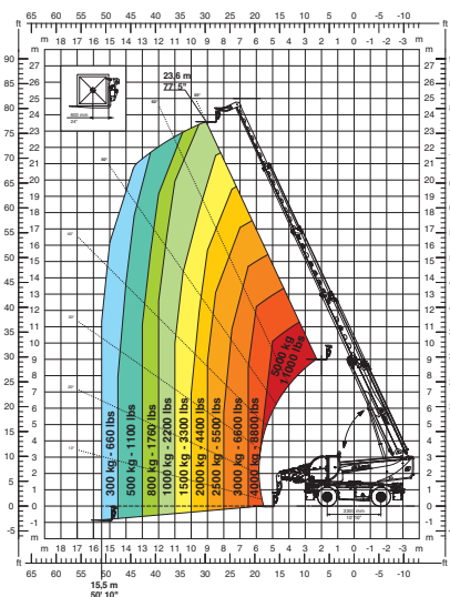
W 3,5 Treuil 3,5 tonnes
