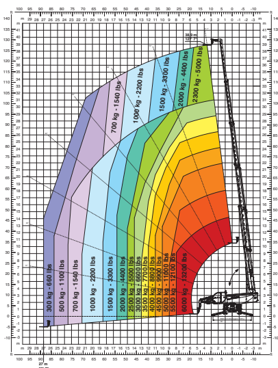
H 6 Crochet 6 tonnes
