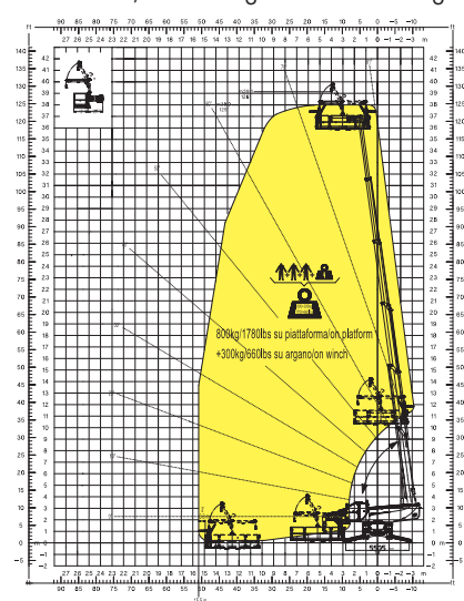
REP 8.2-4,7 W0,3 Nacelle 4,7 m 800 kg avec treuil 300 kg
