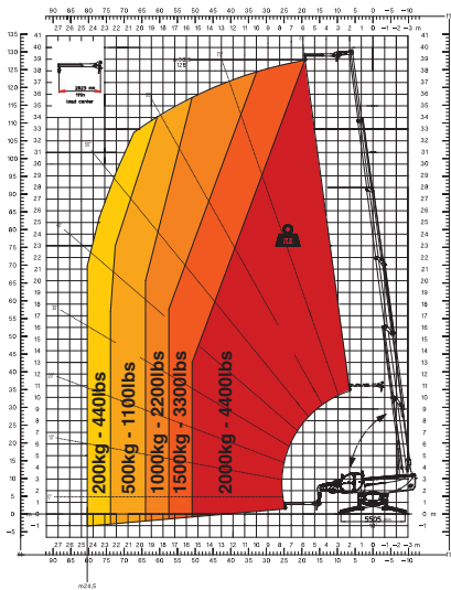
J 2000 Potence 2.000 kg
