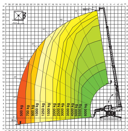
ABAQUE DE CHARGES SUR STABILISATEURS DÉPLOYÉS 360°
