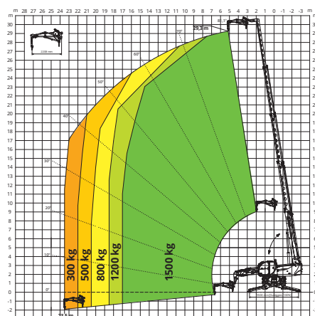
POTENCE AVEC TREUIL 1 500 kg
