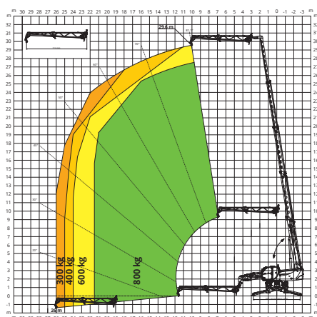
POTENCE AVEC TREUIL 800 kg
