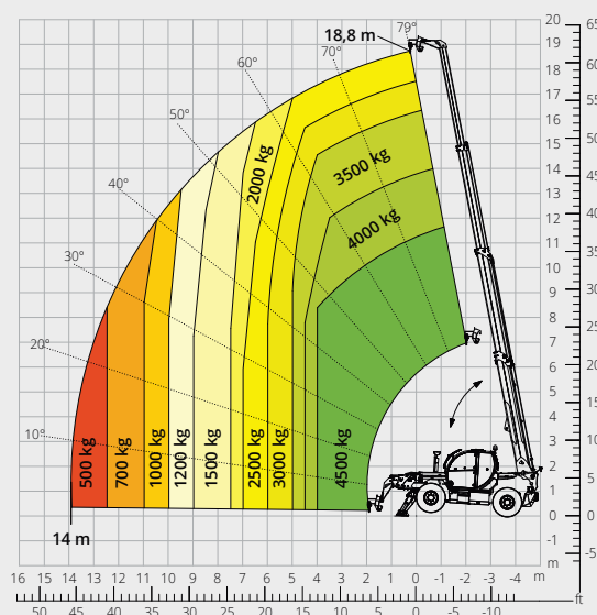
Abaque de charge avec CROCHET 5 000 kg ATT-05-014
