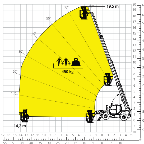
Abaque de charge avec PANIER NACELLE 450 kg POUR MINES ATT-01-027
