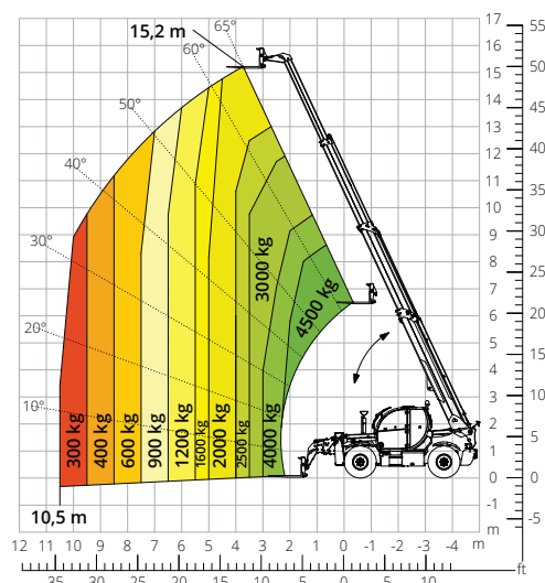
Abaque de charge avec TREUIL 5 000 kg ATT-02-019
