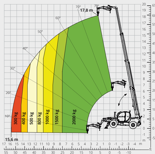
Abaque de charge avec CROCHET 5 000 kg ATT-05-014
