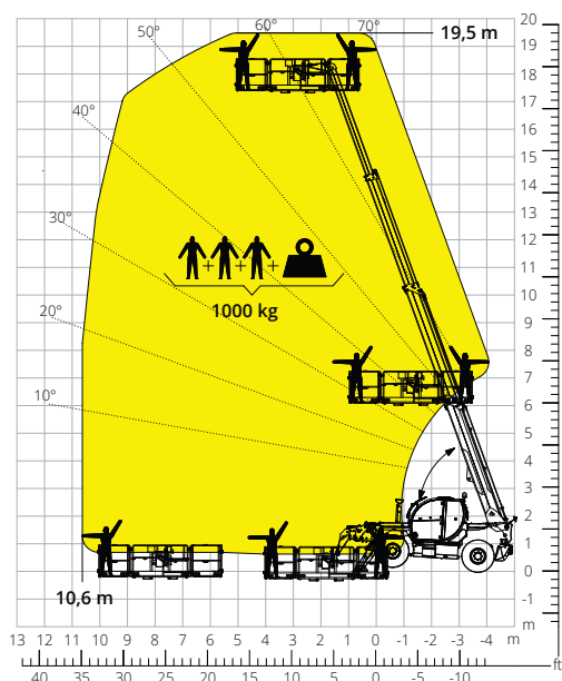
Abaque de charge avec PANIER NACELLE EXTENSIBLE ROTATIF 1 000 kg ATT-01-016
