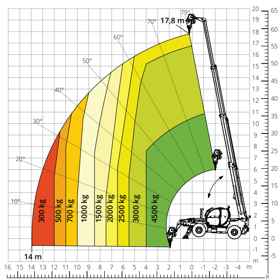
Abaque de charge avec TREUIL 5 000 kg ATT-02-019
