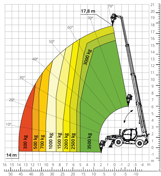
Abaque de charge avec TREUIL 3 500 kg ATT-02-002
