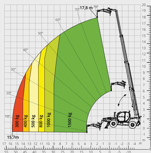
Abaque de charge avec POTENCE 2 000 kg ATT-04-013
