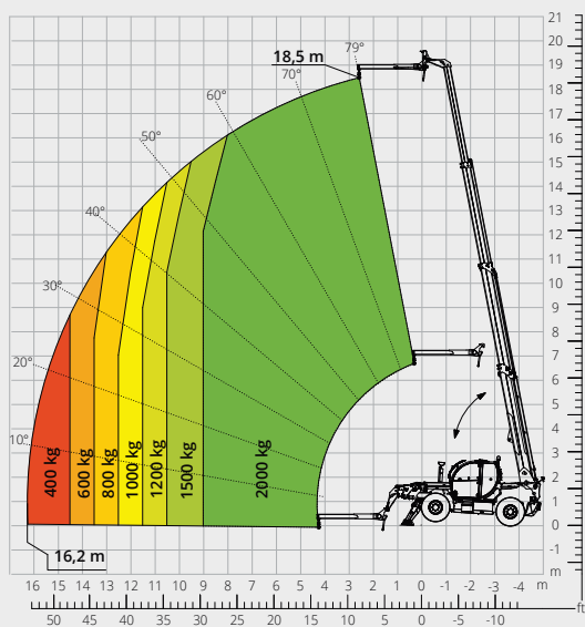
Abaque de charge avec POTENCE 2 000 kg ATT-04-013
