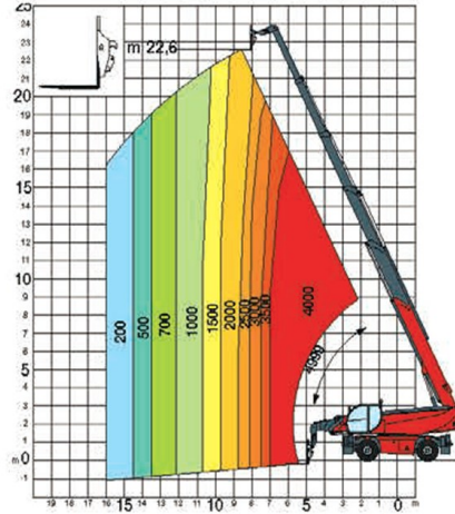
W 5 Winch 5 ton
