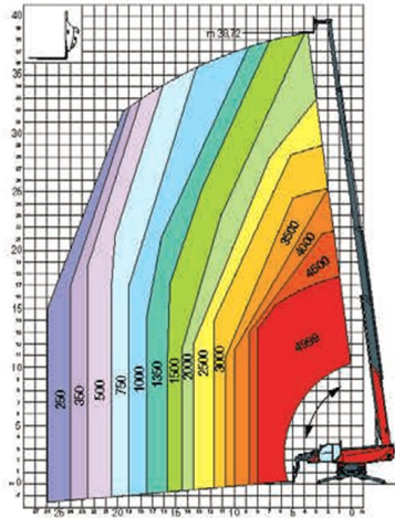
W 3,5 Winch 3,5 ton
