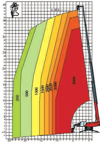
W 3,5 Winch 3,5 ton
