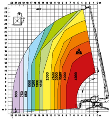
W 3,5 crochet 3,5 tonnes
