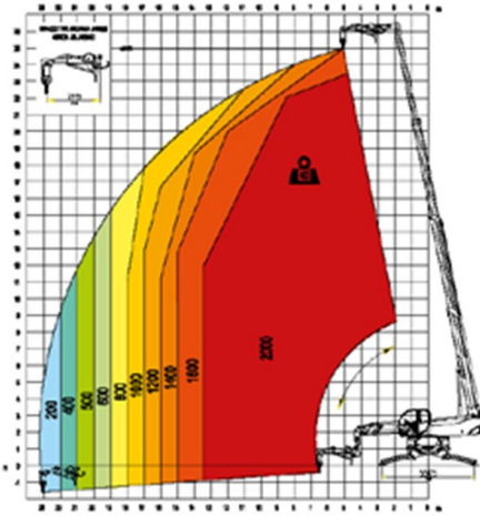
REP 10.2-4,7 nacelle extensible rotative 1000kg
