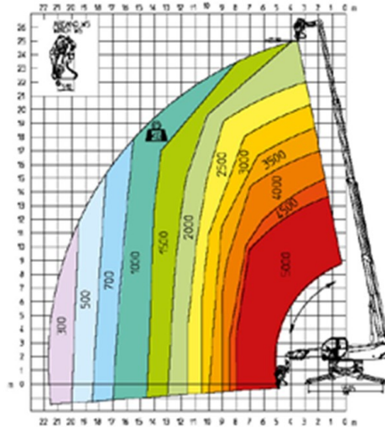
JW 1500 potence avec treuil 1.500
