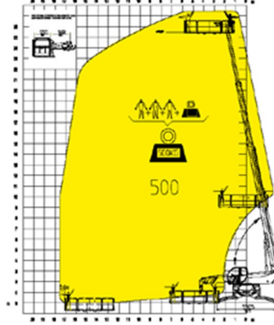
TP 2.10 Plateforme télescopique TP 2.10
