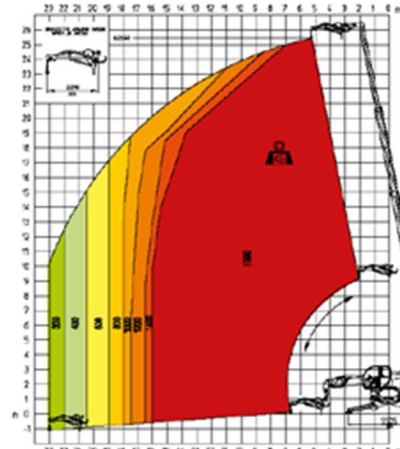
JW 1500 potence avec treuil 1.500
