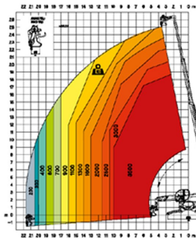
JW 800 potence avec treuil 800
