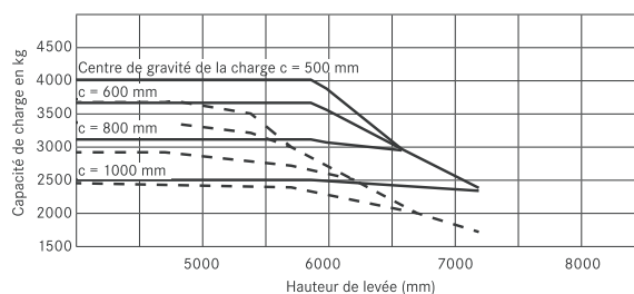
RX 60-40 avec mât triplex
