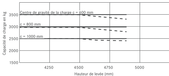
RX 60-35/600 avec mât télescopique
