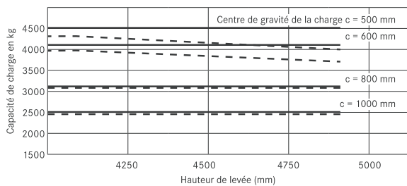
RX 60-45 avec mât télescopique
