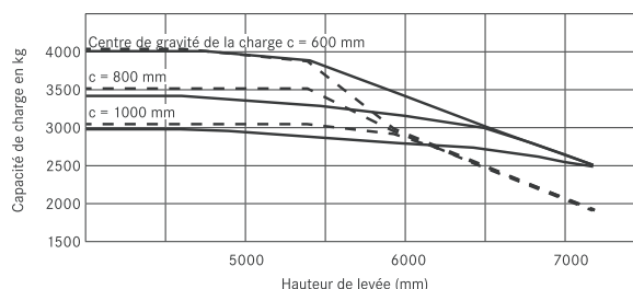
RX 60-40/600 avec mât triplex
