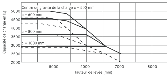
RX 60-50 avec mât triplex
