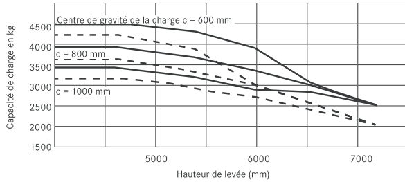
RX 60-45/600 avec mât triplex
