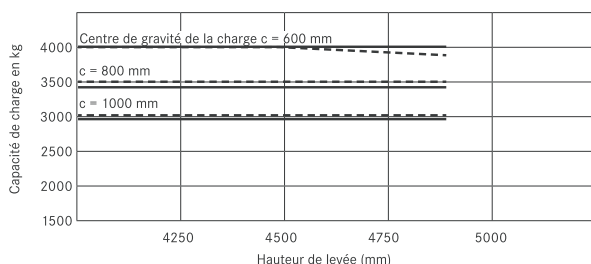
RX 60-40/600 avec mât télescopique
