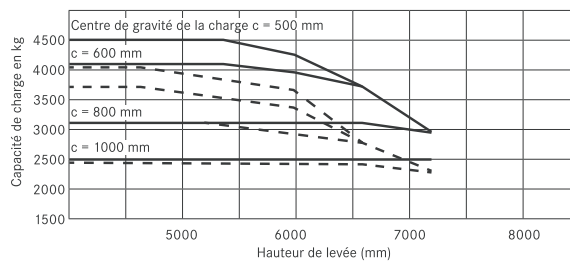
RX 60-45 avec mât triplex/pneus jumelés
