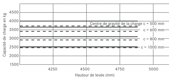
RX 60-40 avec mât télescopique
