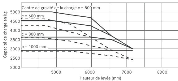
RX 60-50 avec mât triplex/pneus jumelés
