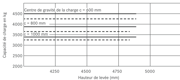
RX 60-45/600 avec mât télescopique
