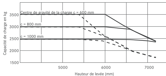
RX 60-35/600 avec mât triplex
