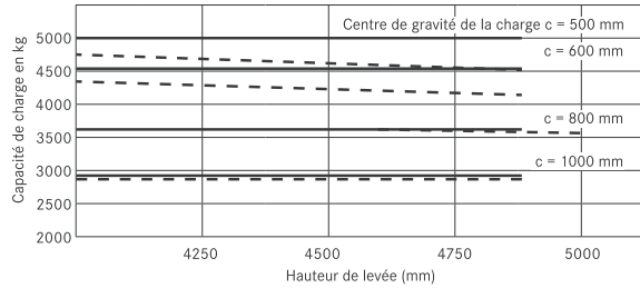
RX 60-50 avec mât télescopique
