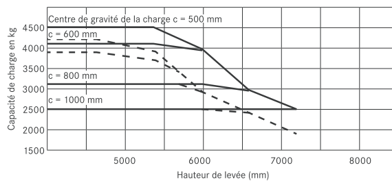
RX 60-45 avec mât triplex
